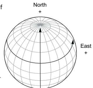
Figure 21.1 Latitude and longitude in decimal degrees
