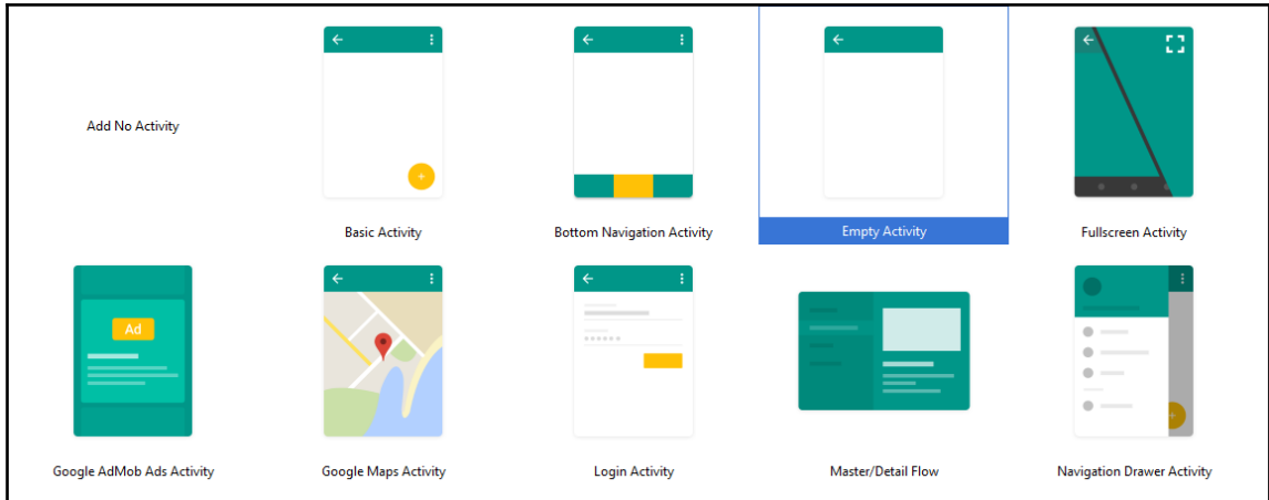
Project templates
