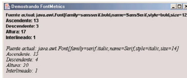
Figura 28.12 Cómo obtener información sobre la métrica de una fuente. (Parte 2 de 2.)
