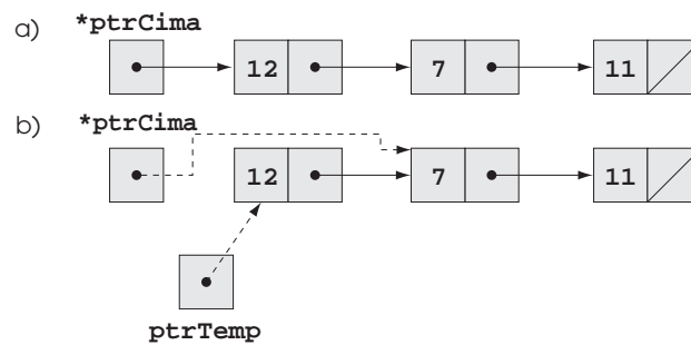
Figura 12.11 Operación pop (sacar).
