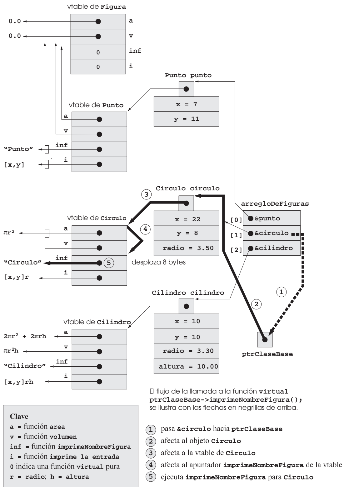
Figura 20.2 Flujo de control de una llamada a una función virtual.
