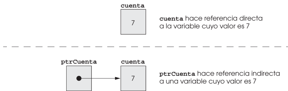
Figura 7.1 Referencias directa e indirecta a una variable.
