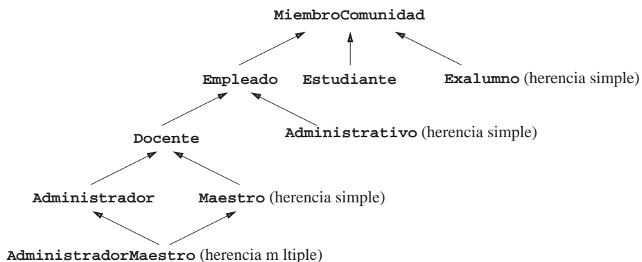
Figura 19.2 Jerarquía de herencia para los miembros de la comunidad universitaria.
