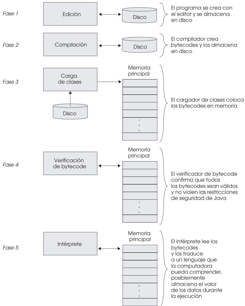
Figura 24.1 Un típico ambiente de Java.
