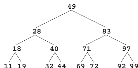
Figura 12.22 Un árbol binario de búsqueda con 15 nodos.
