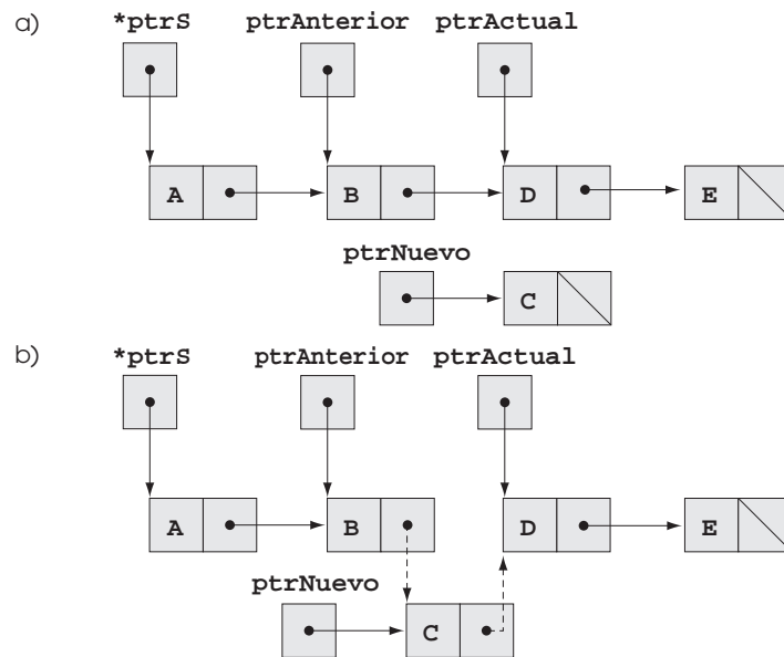
Figura 12.5 Inserción ordenada de un nodo en una lista.
