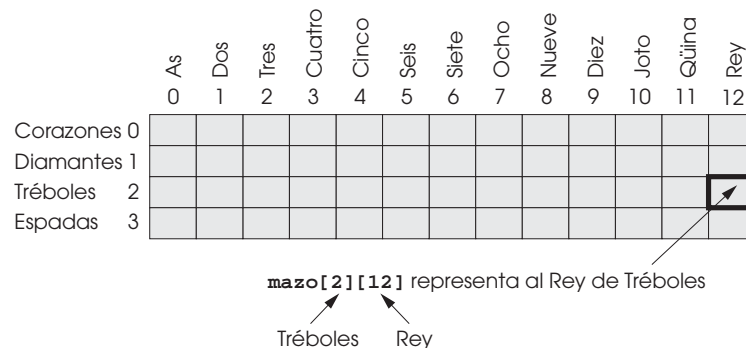
Figura 7.23 Arreglo con dos subíndices que representa un mazo de cartas.
