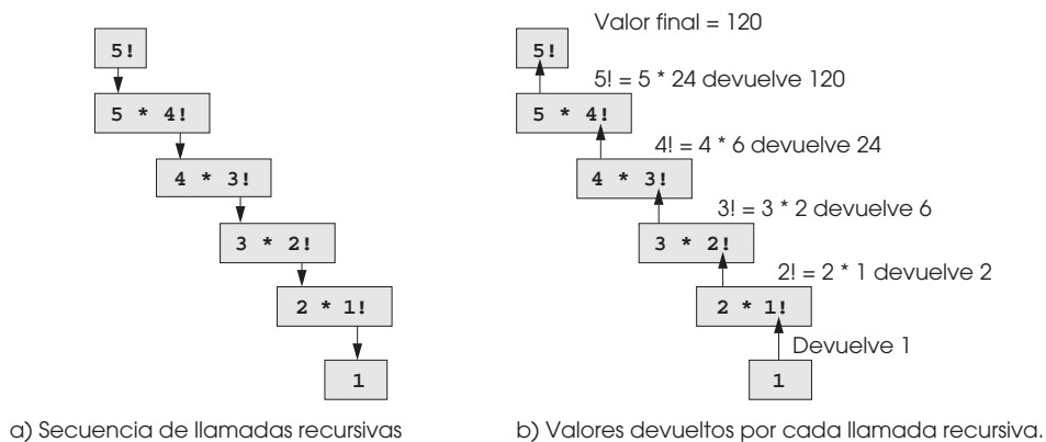
Figura 5.13 Evaluación recursiva de 5!
